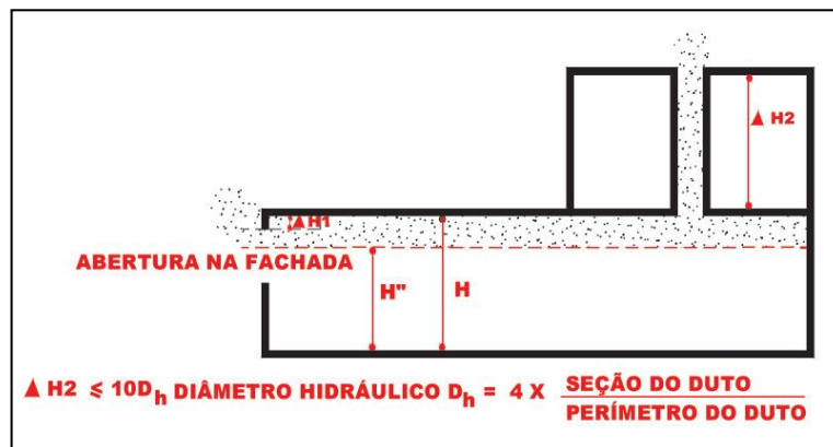
Figura 17 – Diâmetro hidráulico
