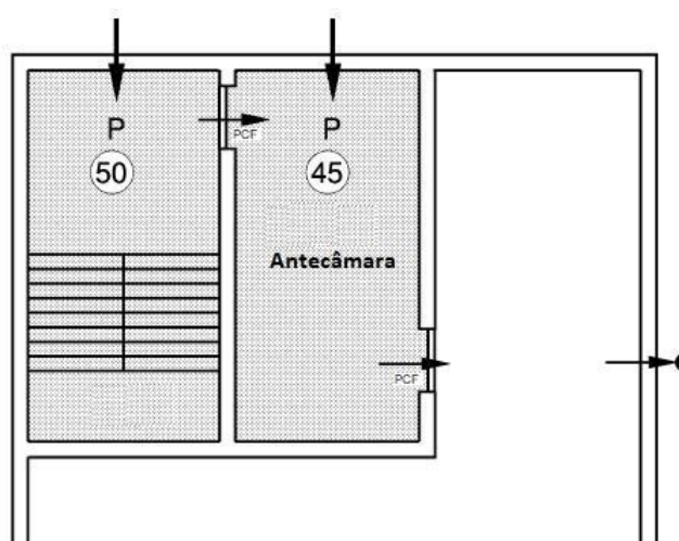
Figura 4 – Pressurização de Antecâmara com insuflação Independente
