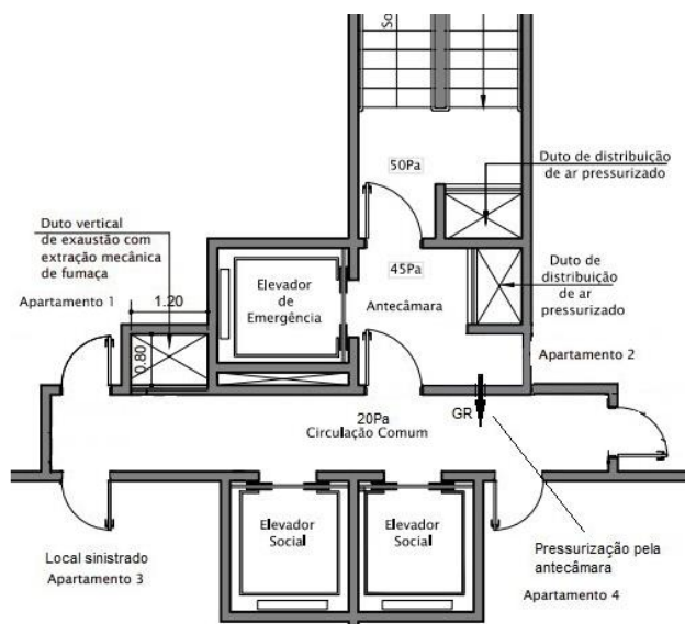
Figura 11 - Equilíbrio de diferencial de pressão
