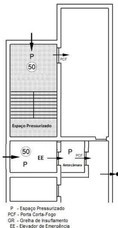
Figura 7 – Pressurização de Antecâmara do Elevador de Emergência a partir do poço do elevador
