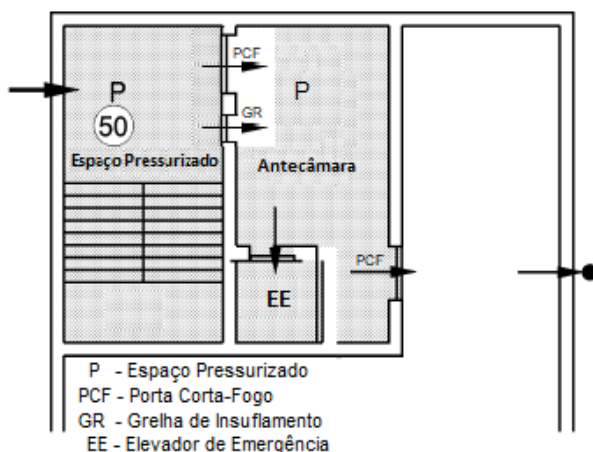
Figura 5 – Pressurização de Antecâmara do Elevador de Emergência contígua a Escada
