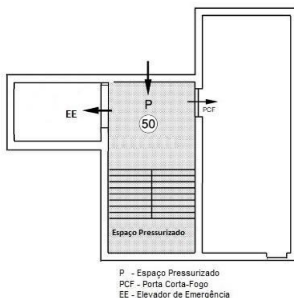
Figura 8 – Pressurização do acesso ao Elevador de Segurança no patamar da Escada Pressurizada
