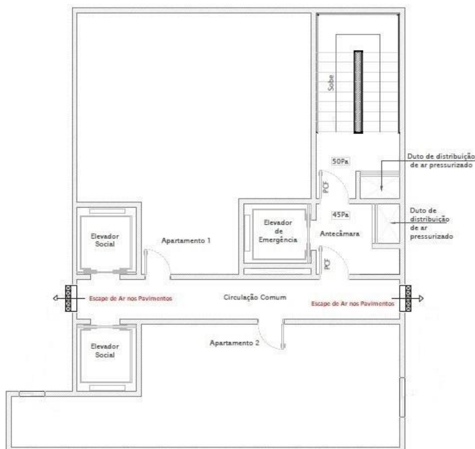
Figura 10 – Escape de ar nos pavimentos
