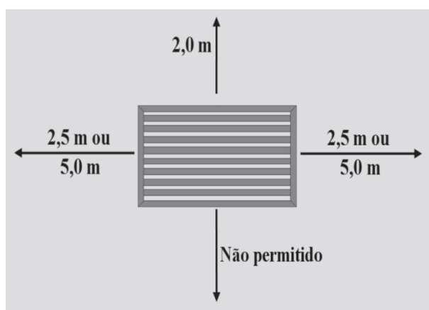
Figura 9 – Distâncias mínimas de aberturas à tomada de ar.
