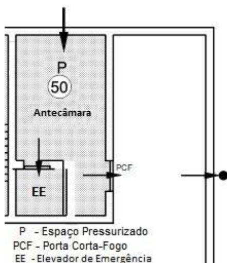
Figura 6 – Pressurização de Antecâmara do Elevador de Emergência
