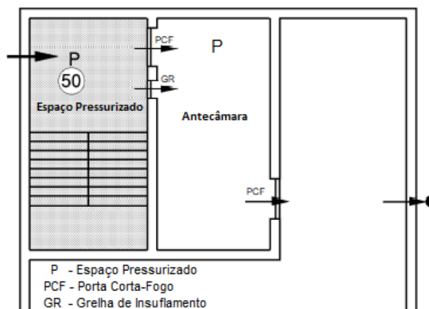
Figura 3 – Pressurização de Antecâmara com insuflação na Escada.
