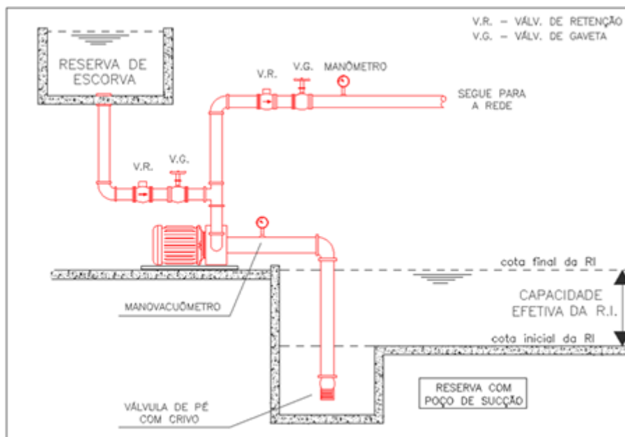
Figura C-3 – Exemplo de afogamento de bomba de incêndio
