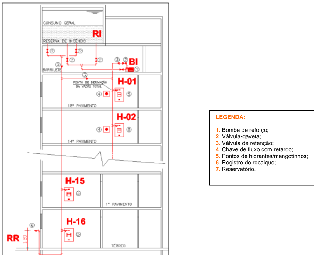
Figura C-6 – Esquema de instalação de bomba de reforço abastecendo os pontos de hidrante ou mangotinhos mais desfavoráveis considerados no cálculo (prumada específica)
