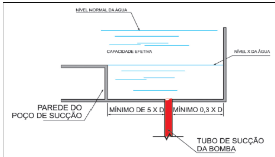
Figura B-3 – Tomada inferior de sucção para bomba fixa
