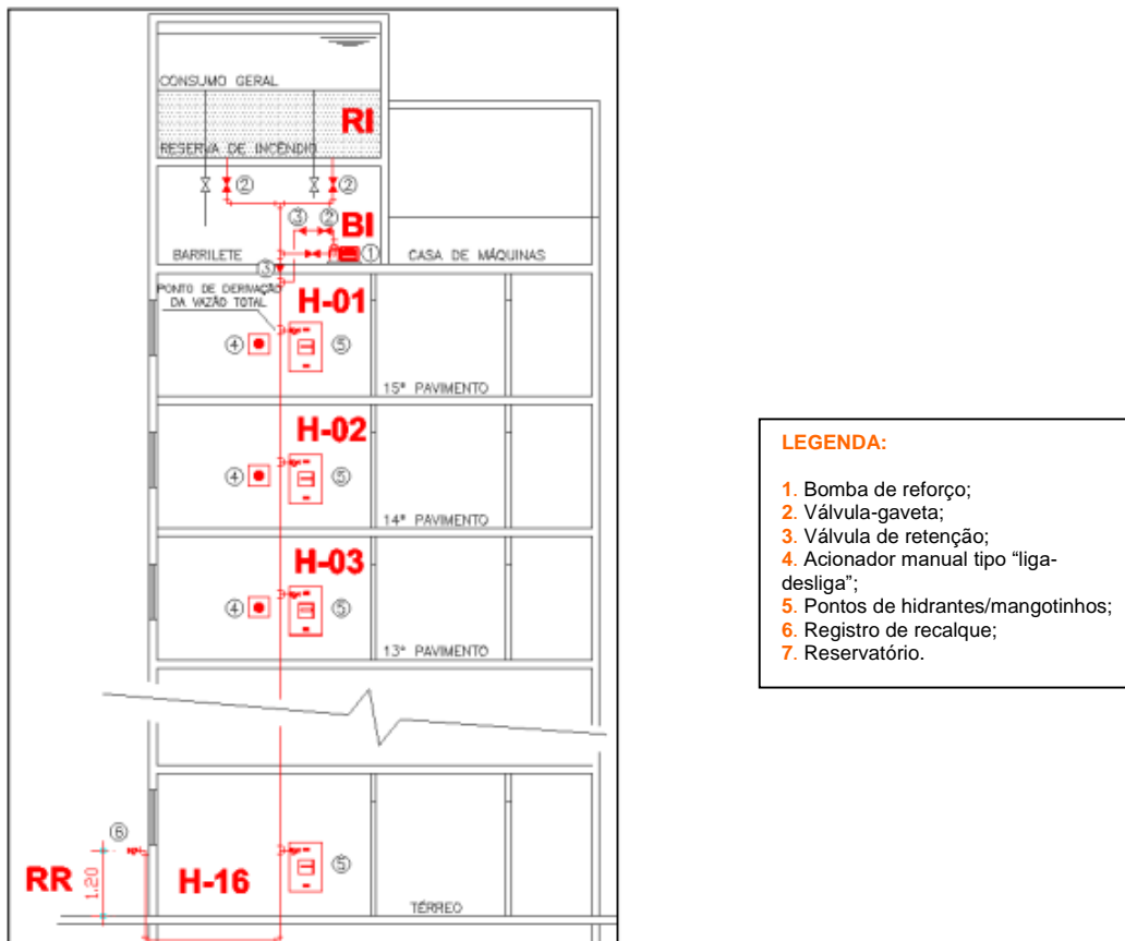
Figura C-5 – Esquema de instalação de bomba de reforço abastecendo os pontos de hidrante ou mangotinhos mais desfavoráveis considerados no cálculo (prumada específica)
