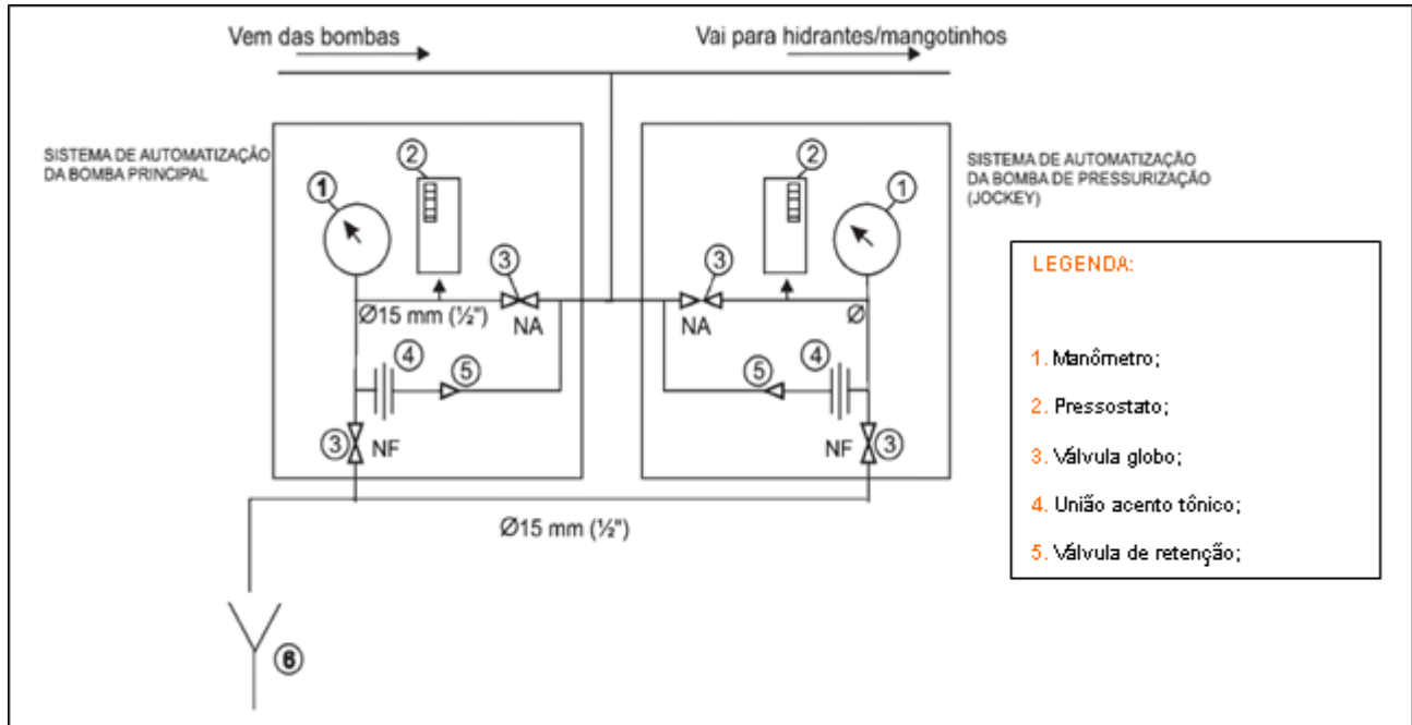
Figura C-2 – Cavalete de automação das bombas fixa e de pressurização
