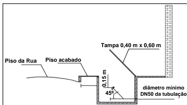
Figura 2 – Dispositivo de recalque no passeio público
