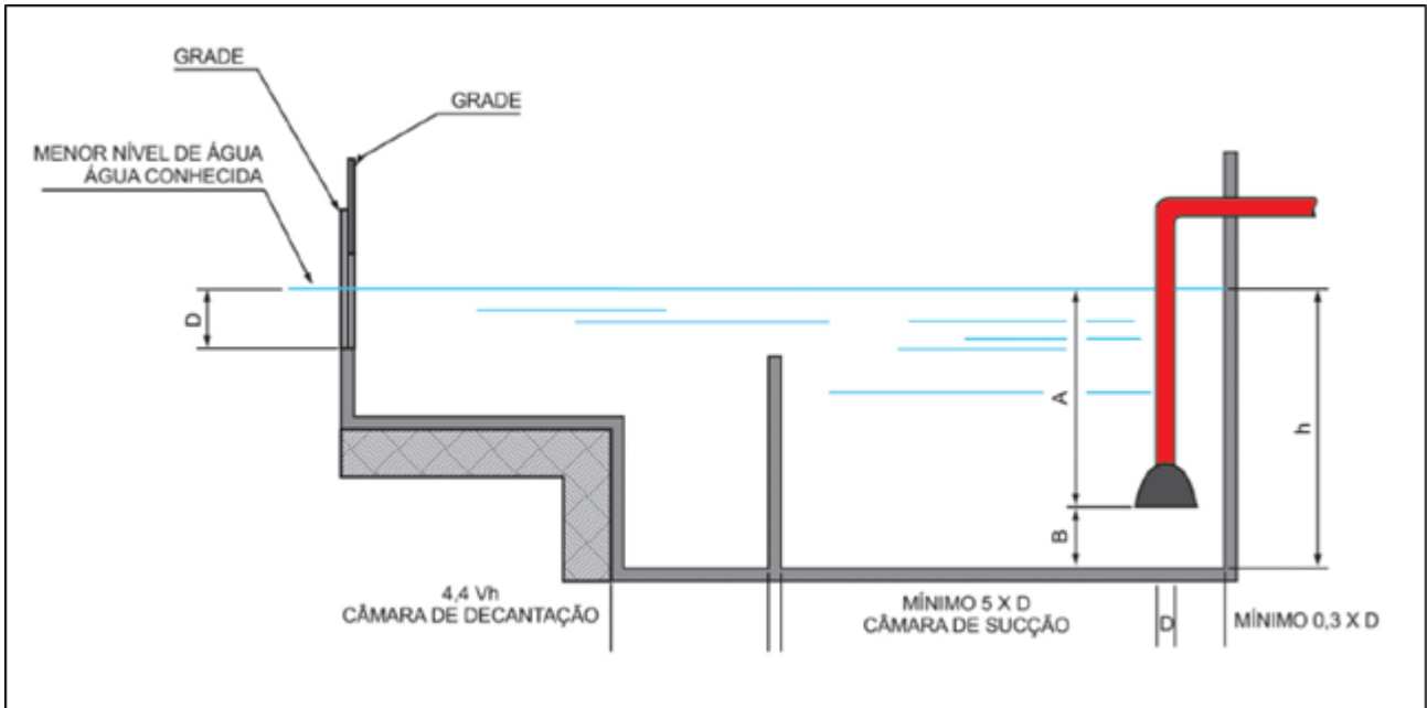
Figura B-4 – Alimentação natural de reservatório por canal
