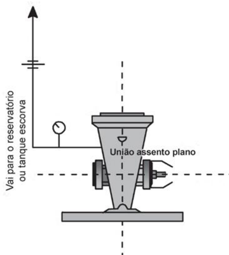
Figura C-7 – Arrefecimento da bomba de incêndio
