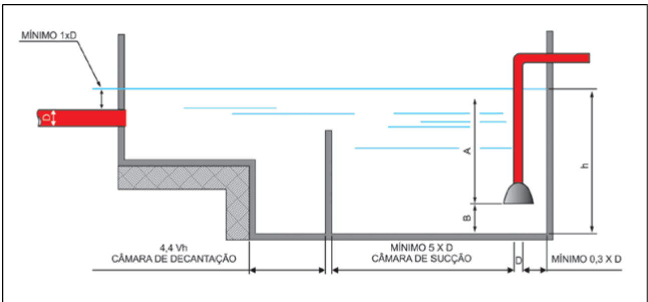
Figura B-5 – Alimentação natural de reservatório por conduto
