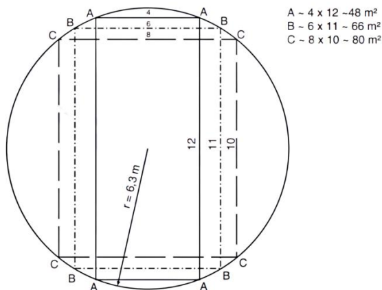
Figura 2 – Cobertura do detector pontual de fumaça em áreas retangulares.
