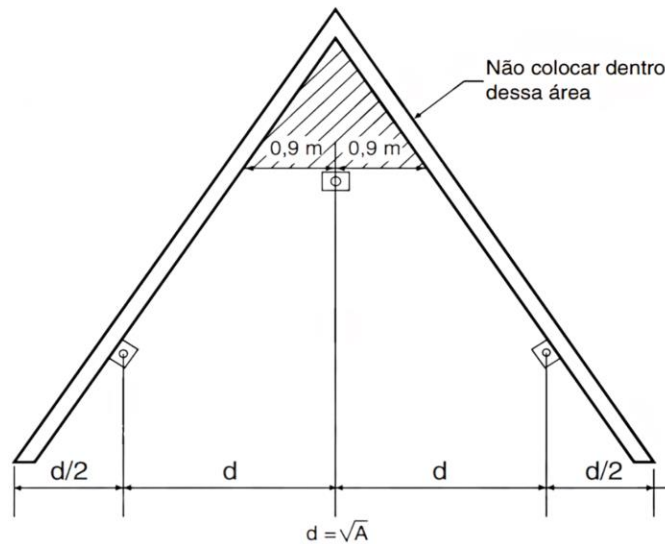
Figura 8 – Distribuição de detectores pontuais de fumaça em planos inclinados, com ventilação na cumeeira.
