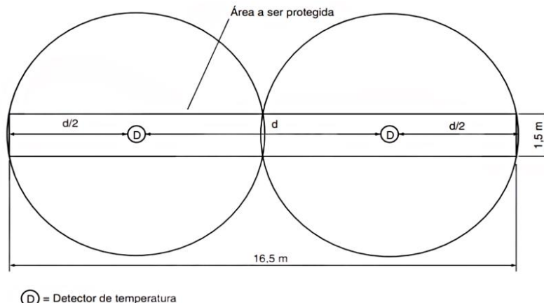
Figura 17 – Distribuição de detectores pontuais de temperatura em área retangular, menor que 36 m 2 .
