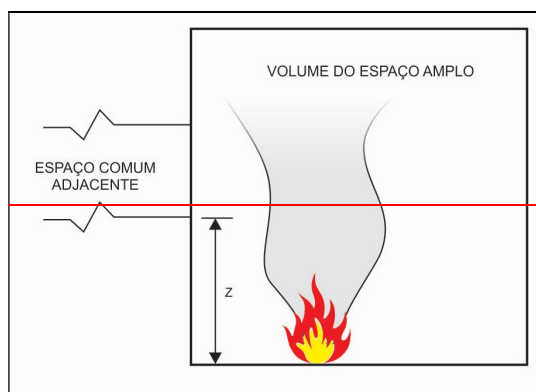
Figura 43 – Coluna de fumaça saindo por aberturas (janelas)
