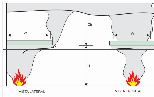
Figura 41 – Coluna de fumaça saindo de um balcão
