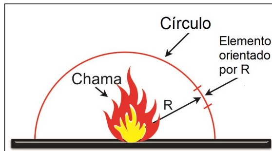
Figura 39 — Distância de separação R
