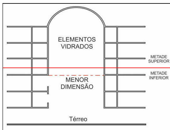
Figura 35 – Fechamento do átrio
