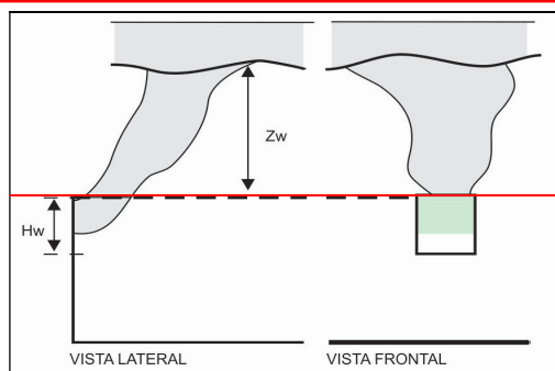
Figura 42 – Coluna de fumaça saindo por aberturas (janelas)
