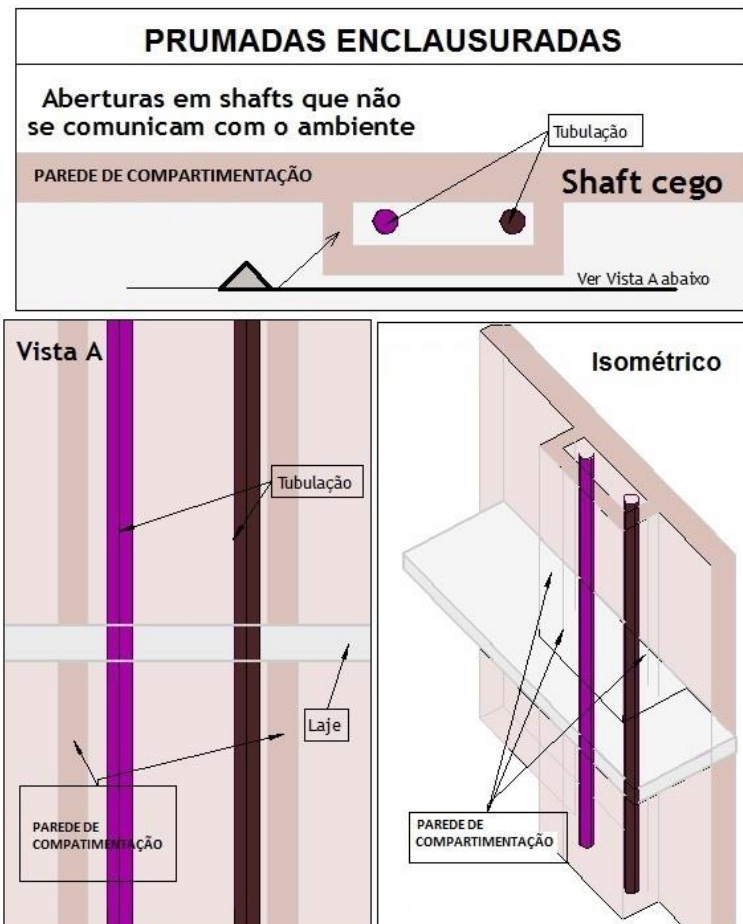
Figura D2 – Prumadas Enclausuradas.
