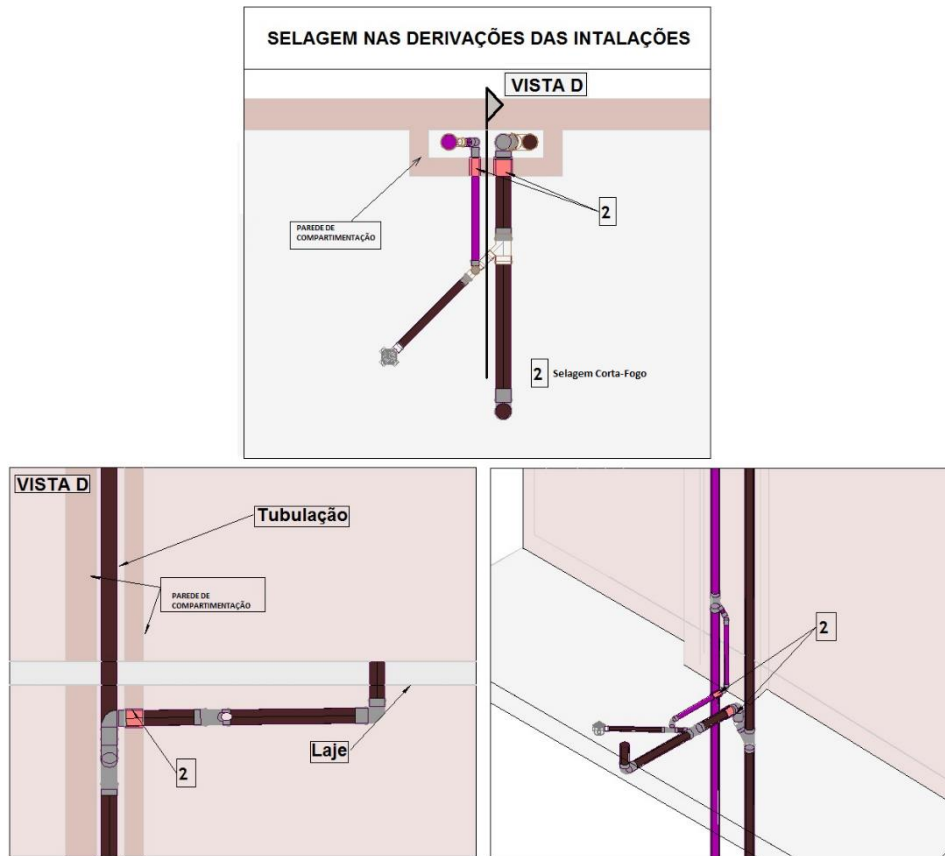
Figura D3 – Selagem nas derivações das instalações.
