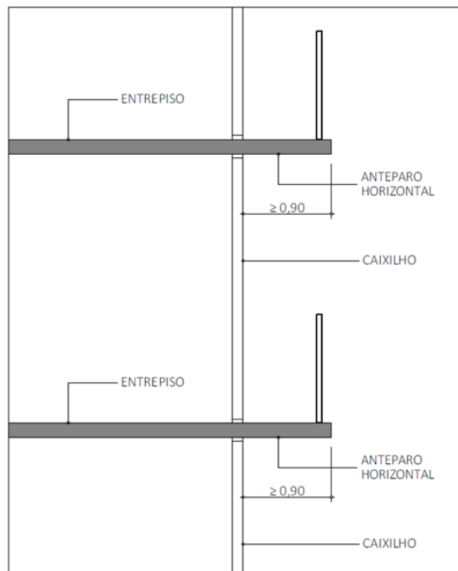
Figura C3 – Modelo de compartimentação com anteparo horizontal.
