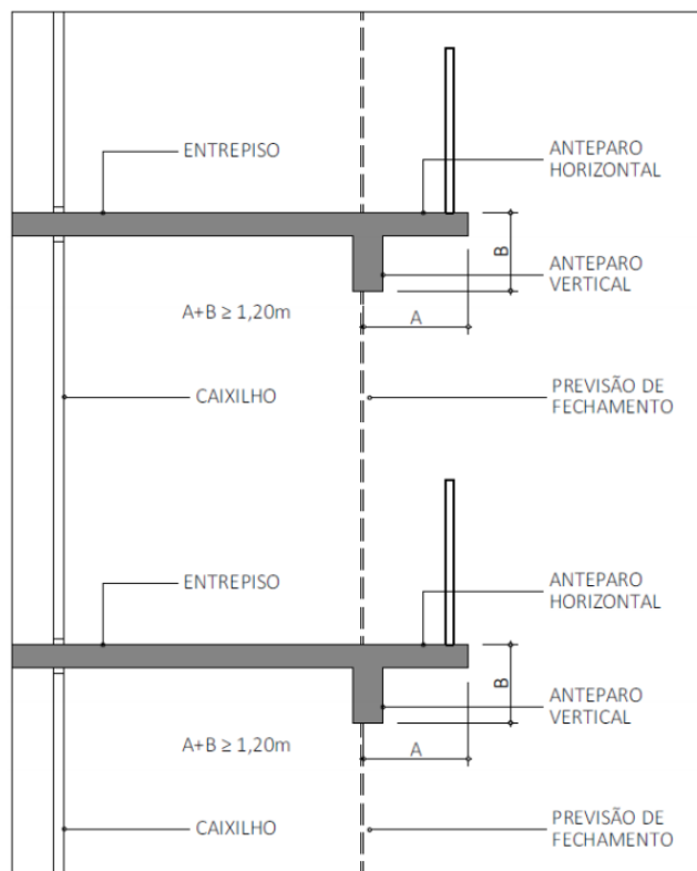
Figura C9 – Modelo de fechamento com vidro.
