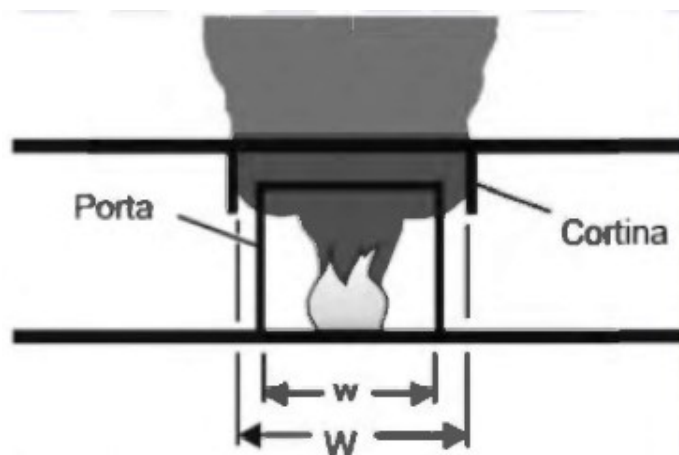
Figura 19 – Vista frontal da porta com cortinas de direcionamento
