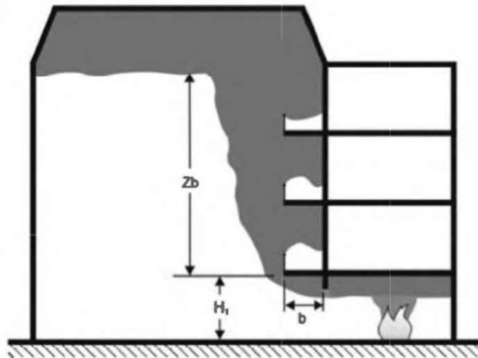
Figura 18 – Extração da coluna de fumaça no mezanino - vista lateral em corte
