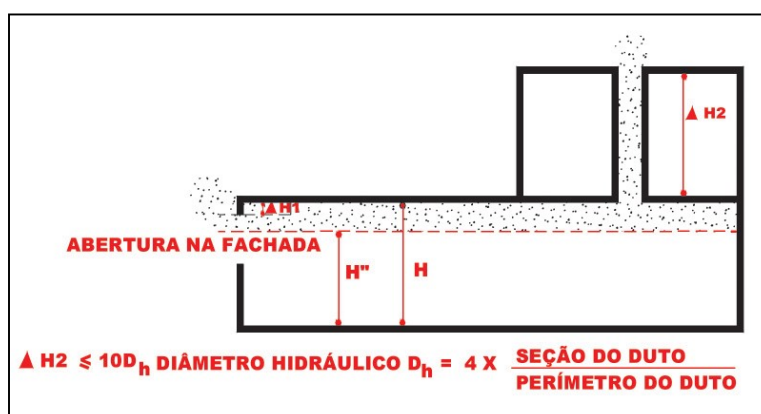
Figura 17 – Diâmetro hidráulico
