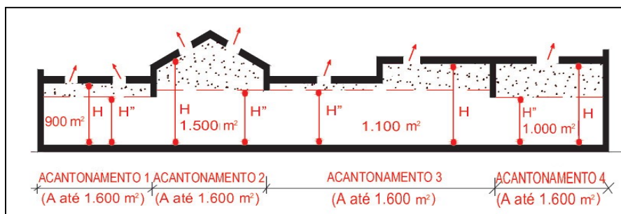
Figura 16 – Altura de referência diversificada por acantonamento
