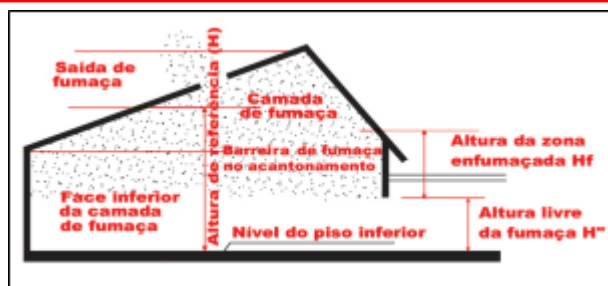
Figura 14 – Altura de referência, livre de fumaça e da zona enfumaçada
