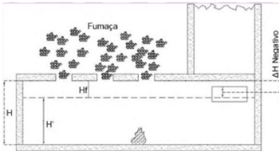
Figura 19 - Extrator instalado abaixo da altura de referência ( \Delta H Negativo)
