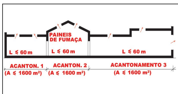
Figura 13 – Divisão em áreas de acantonamento
