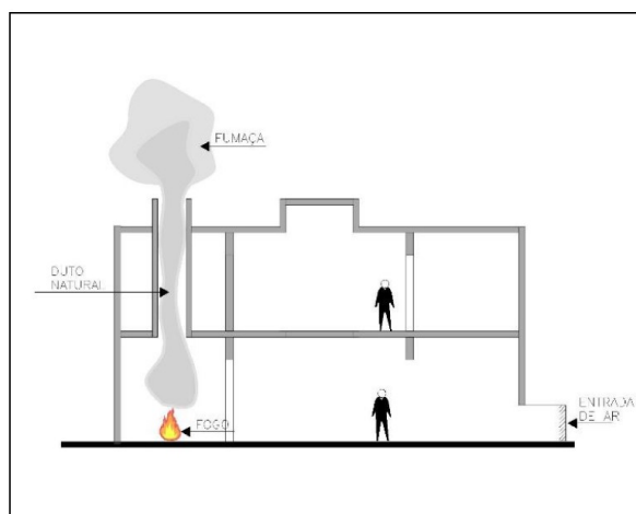
Figura 12 – Exemplo de controle de fumaça por extração natural e entrada de ar natural, por meio de dutos
