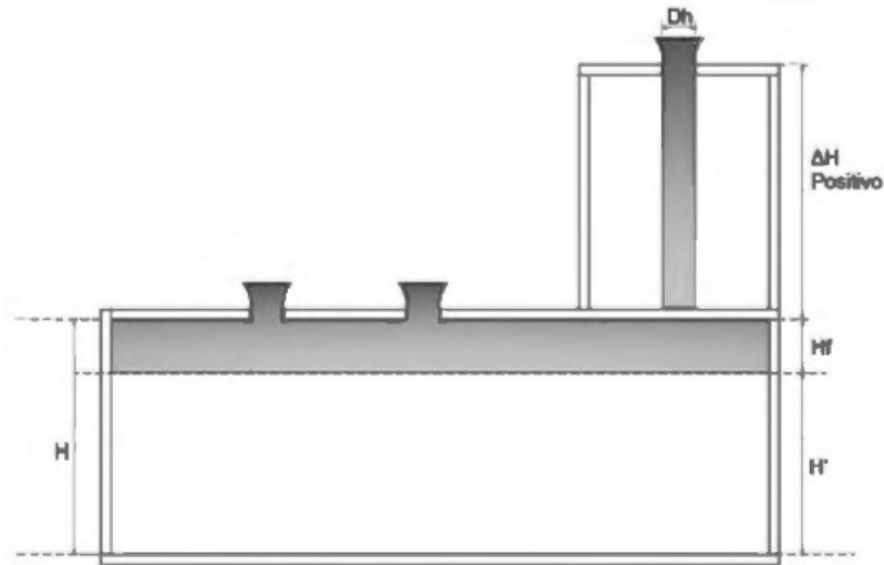
Figura 18 - Extrator instalado acima da altura de referência ( \Delta H positivo)
