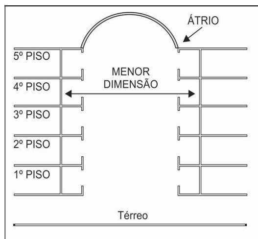
Figura 35 – Modelo 2 de átrios cobertos fechados
