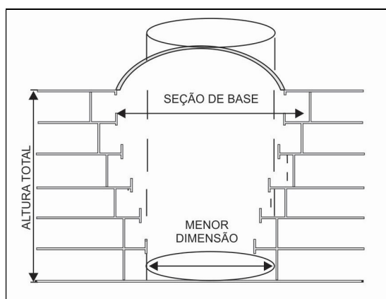
Figura 37 – Dados relativos a um átrio coberto padronizado
