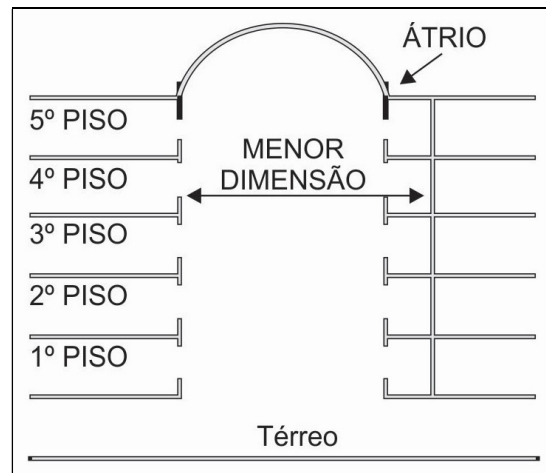
Figura 33 – Átrio coberto aberto
