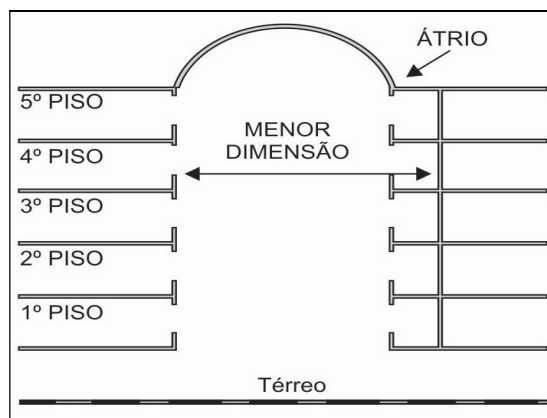
Figura 36 – Átrio considerado aberto de um lado e fechado do outro
