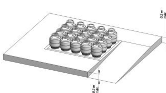
Figura 2 – Exemplo de Área de Armazenamento com Corredor de Circulação Inclinado
