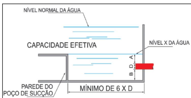
Figura B.2 – Tomada lateral de sucção para bomba fixa
