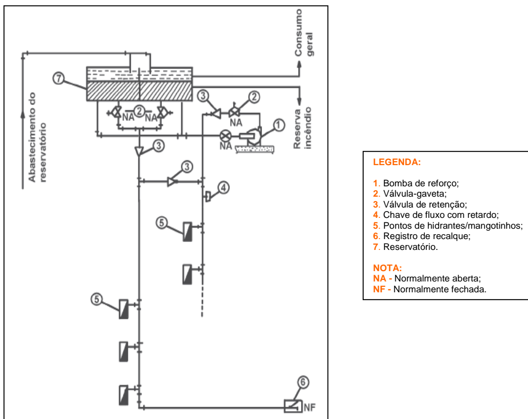
Figura C-5 – Esquema de instalação de bomba de reforço abastecendo os pontos de hidrante ou mangotinhos mais desfavoráveis considerados no cálculo (prumada específica)
