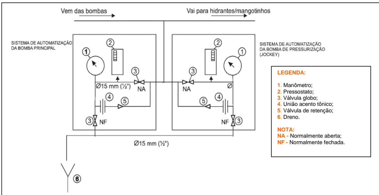
Figura C-3 – Cavalete de automação das bombas fixa e de pressurização
