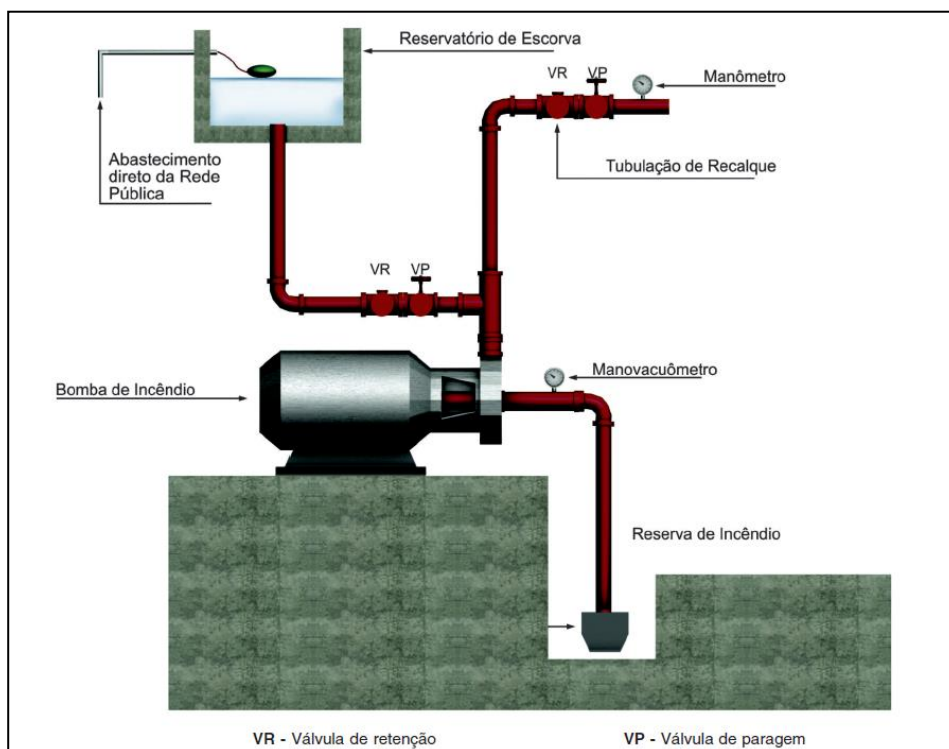
Figura C-2 – Exemplo de afogamento de bomba de incêndio
