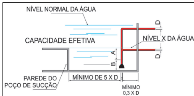
Figura B.1 – Tomada superior de sucção para bomba fixa
