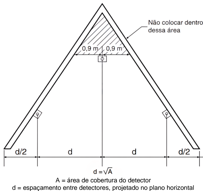
Figura 8 – Distribuição de detectores pontuais de fumaça em planos inclinados, com ventilação na cumeeira.
