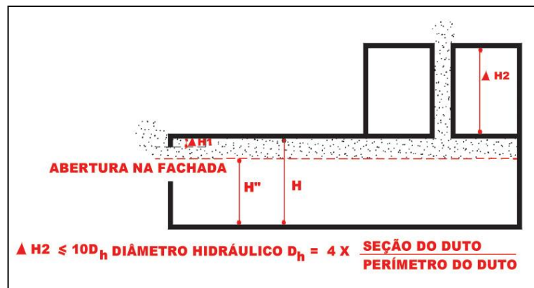
Figura 17 – Diâmetro hidráulico
