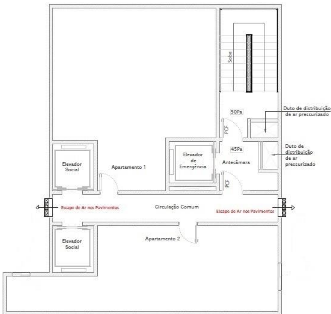
Figura 10 – Escape de ar nos pavimentos
