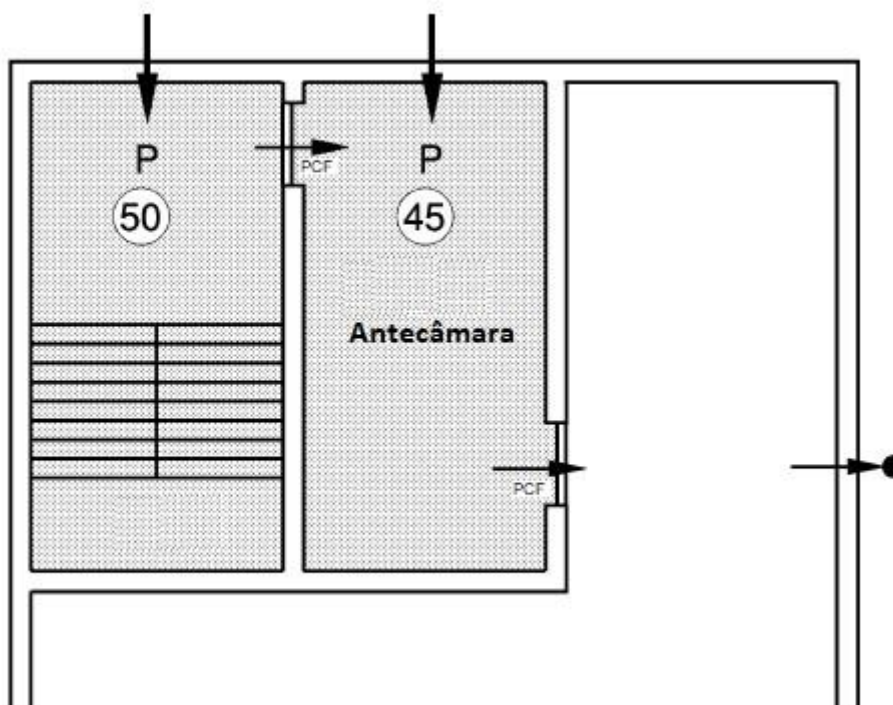
Figura 4 – Pressurização de Antecâmara com insuflação Independente
