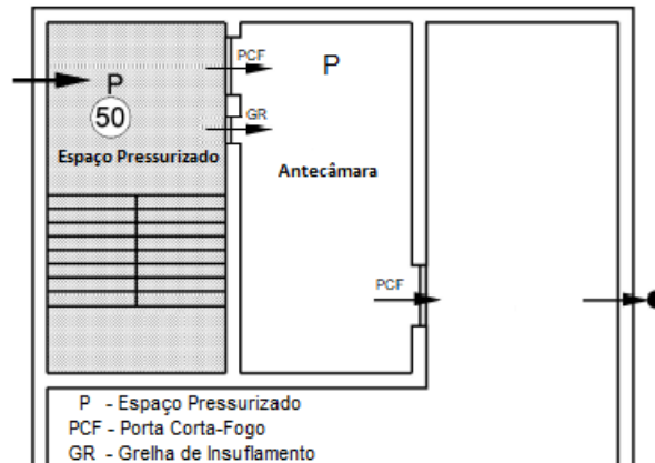
Figura 3 – Pressurização de Antecâmara com insuflação na Escada.
