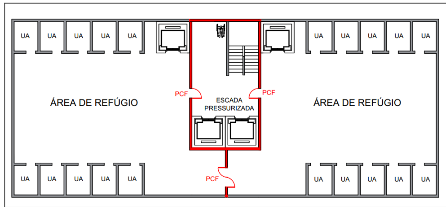
Figura 18 – Exemplos esquemáticos de áreas de refúgio (Ilustrativo).
