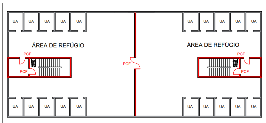
Figura 19 – Exemplos esquemáticos de áreas de refúgio (Ilustrativo).
