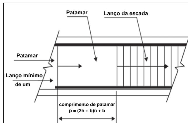
Figura 5 – Lanço mínimo e comprimento de patamar
