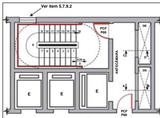
Figura 9 – Escada Enclausurada à Prova de Fumaça com elevador de Emergência (a posição deste é somente exemplificativa) na antecâmara.
