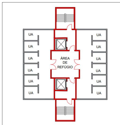
Figura 17 – Exemplos esquemáticos de áreas de refúgio (Ilustrativo).
