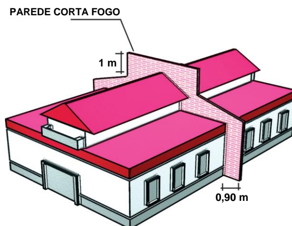
Figura 8 – Parede corta-fogo.
