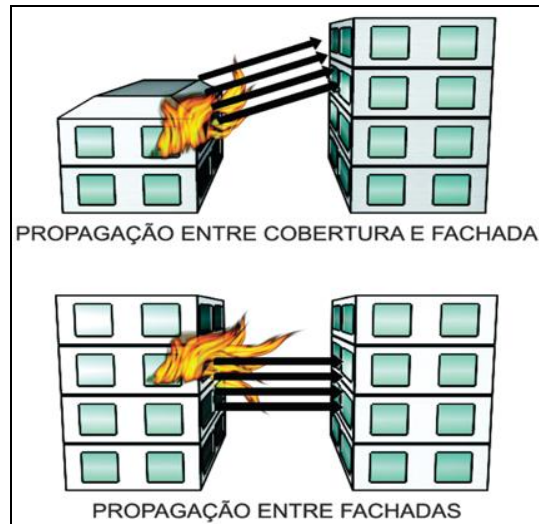
Figura 14 – Isolamento por distância de afastamento
