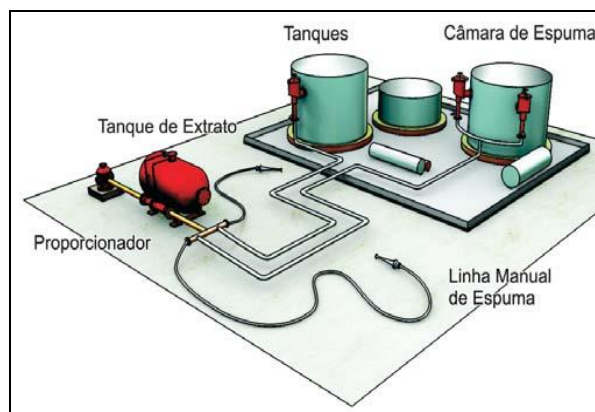
Figura 48 – Sistema semifixo
