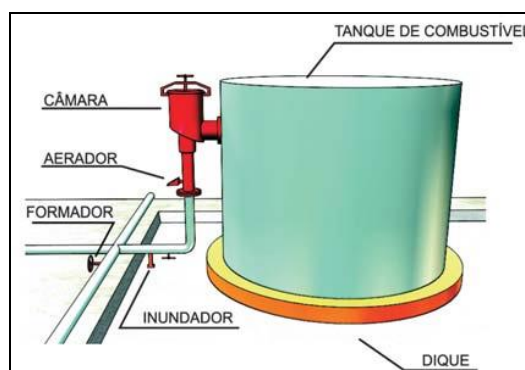
Figura 49 – Detalhe de câmara de espuma
