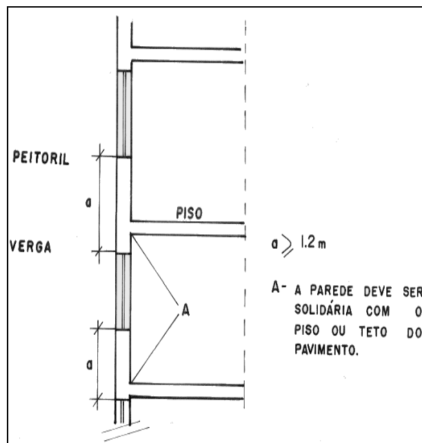
Figura 17 – Distância de afastamento entre verga e peitoril
