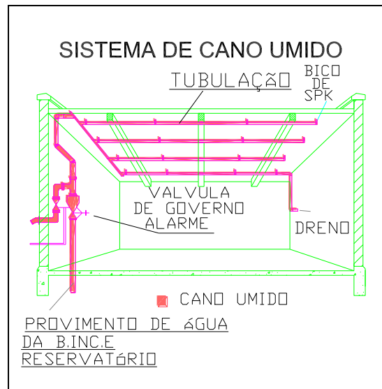
Figura 45 – Esquema de uma rede de chuveiro automático
