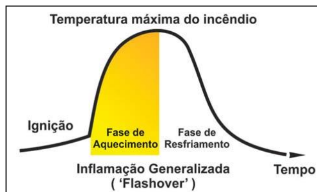
Figura 4 – Curva temperatura tempo de um incêndio
