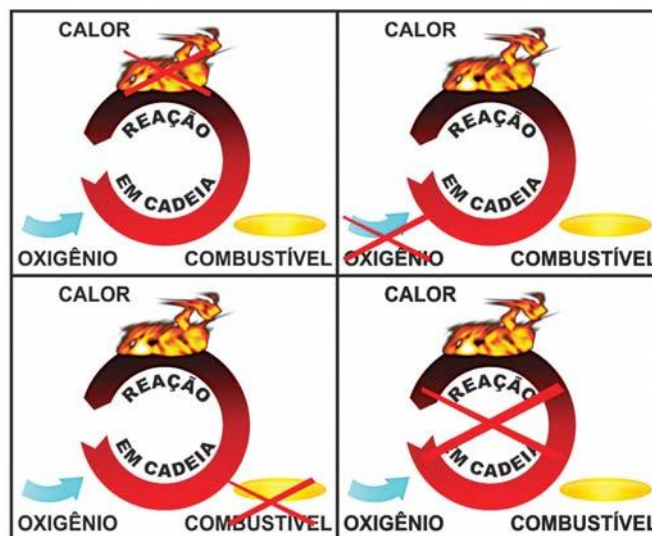
Figura 3 – Mecanismo de extinção do fogo
