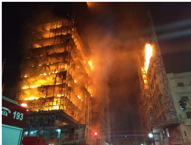
Figura 13 – Propagação por radiação, convecção e condução (Fonte: Corpo de Bombeiros SP)
