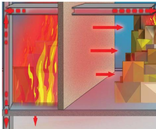
Figura 6 – Propagação por condução (Fonte: Escola Nacional de Bombeiros, Fenomenologia da Combustão e extintores, Volume VII)
