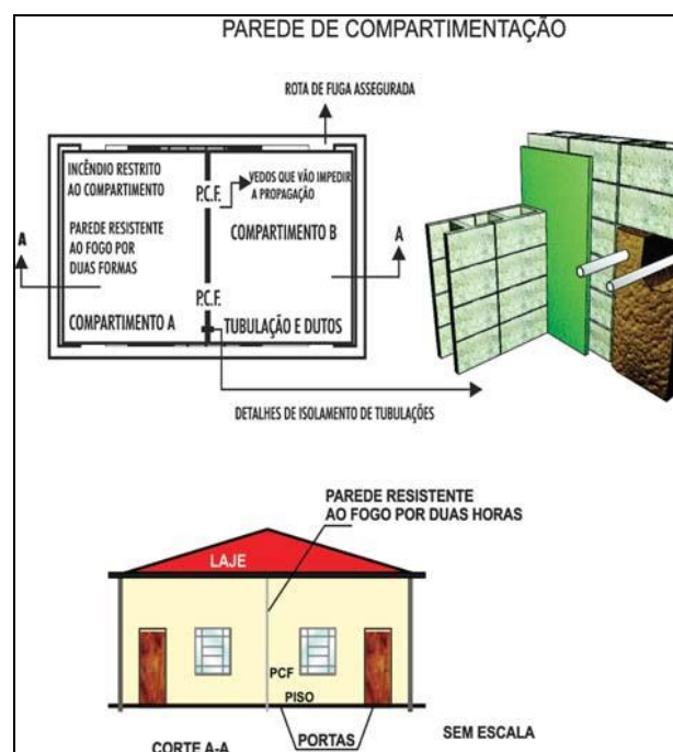
Figura 16 – Detalhes de parede de compartimentação
