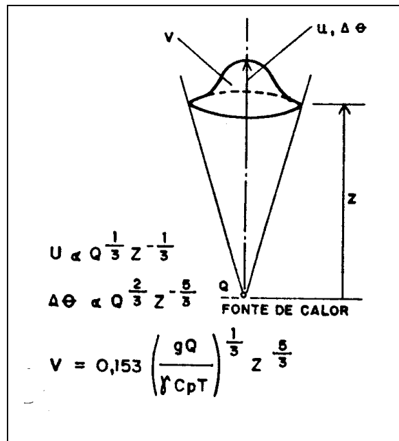
Figura 10 – Plume de fumaça
