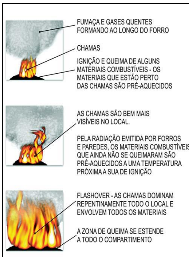
Figura 21 – Evolução da propagação nos materiais
