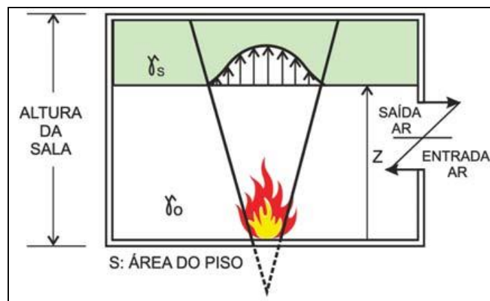
Figura 11 – Processo de formação de gases e fluxo básico do ar
