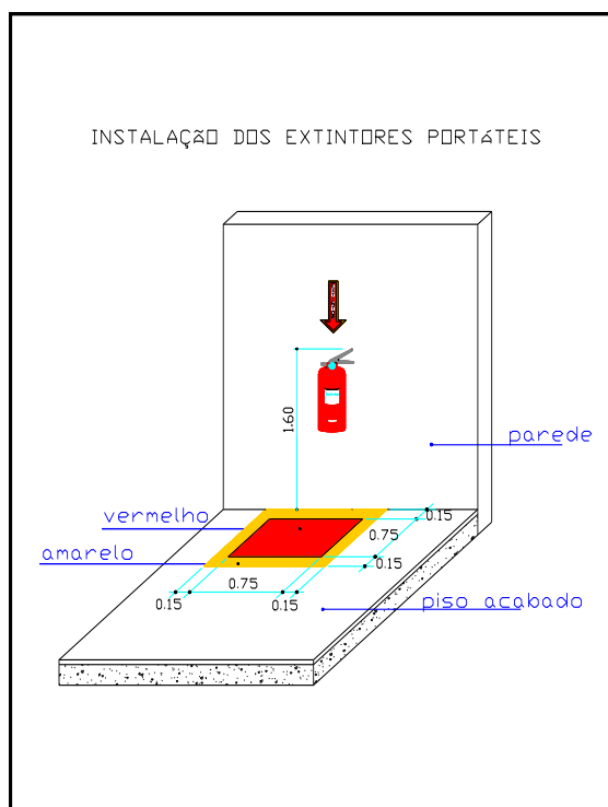
Figura 38 – Detalhe de instalação de extintores em áreas sujeitas à obstrução
