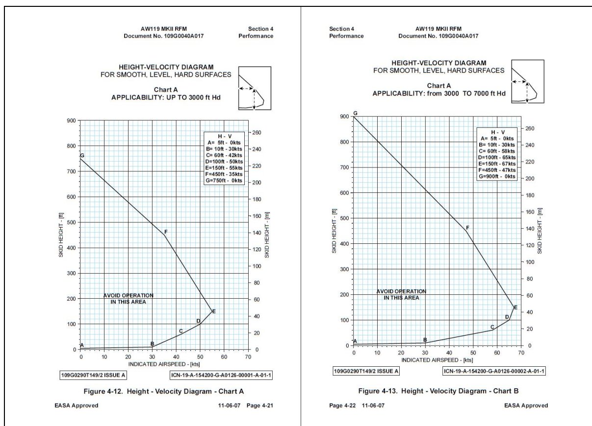
Figura 1- Diagramas altura-velocidade
