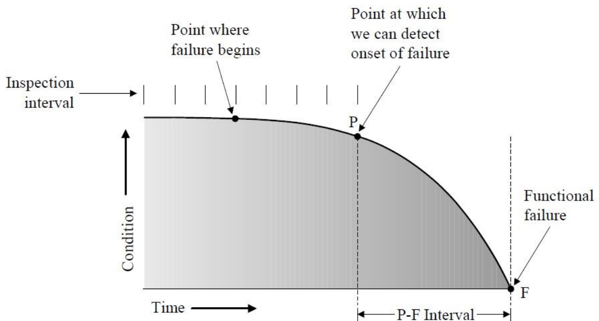
Figura 3- Diagrama P-F
