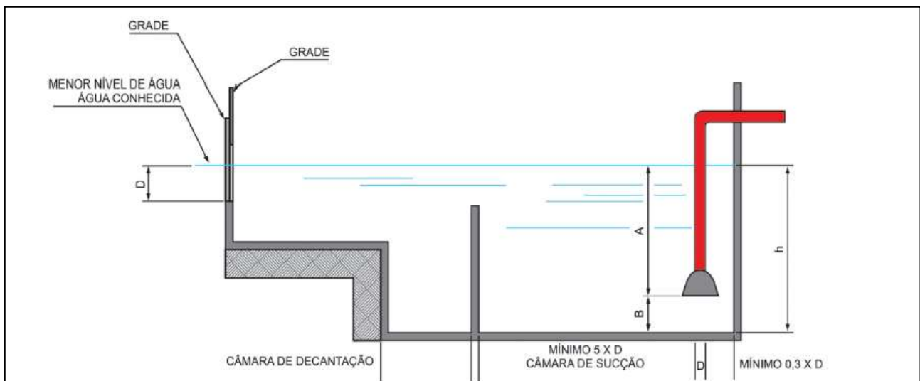
Figura B.4 – Alimentação natural do reservatório de incêndio
