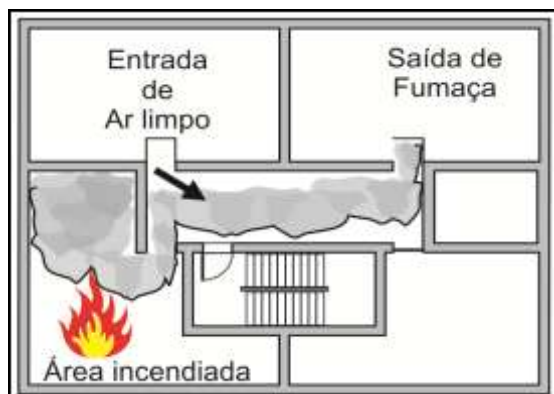
Figura 24 – Extração mecânica
