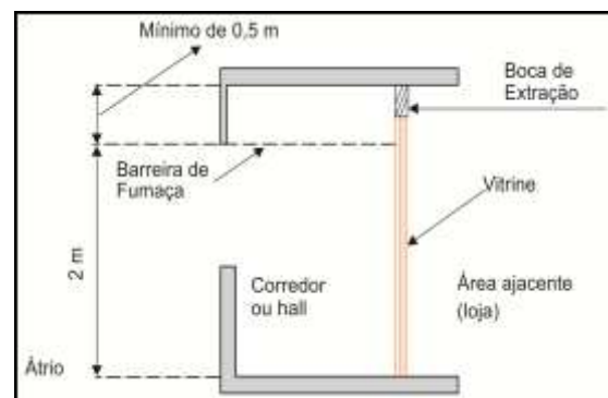
Figura 8 – Detalhe de barreira de fumaça - corte
