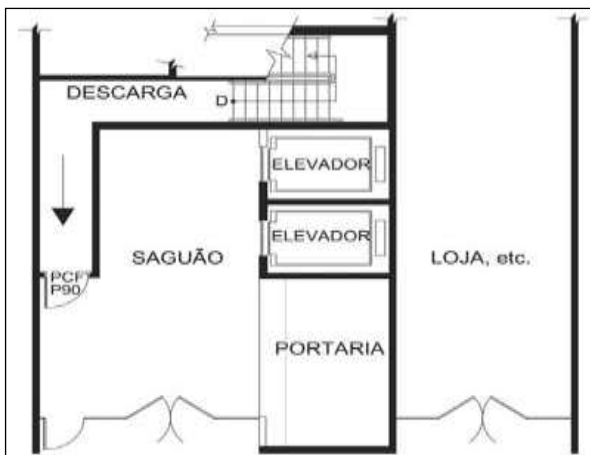
Figura 18 – Descarga através de hall térreo não-enclausurado
