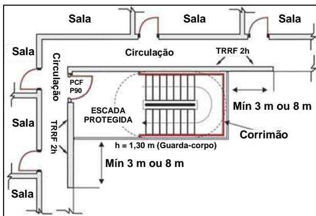
Figura 13 – Escada aberta externa
