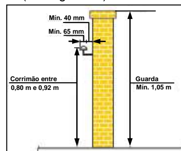
Figura 14 – Dimensões de guardas e corrimãos
