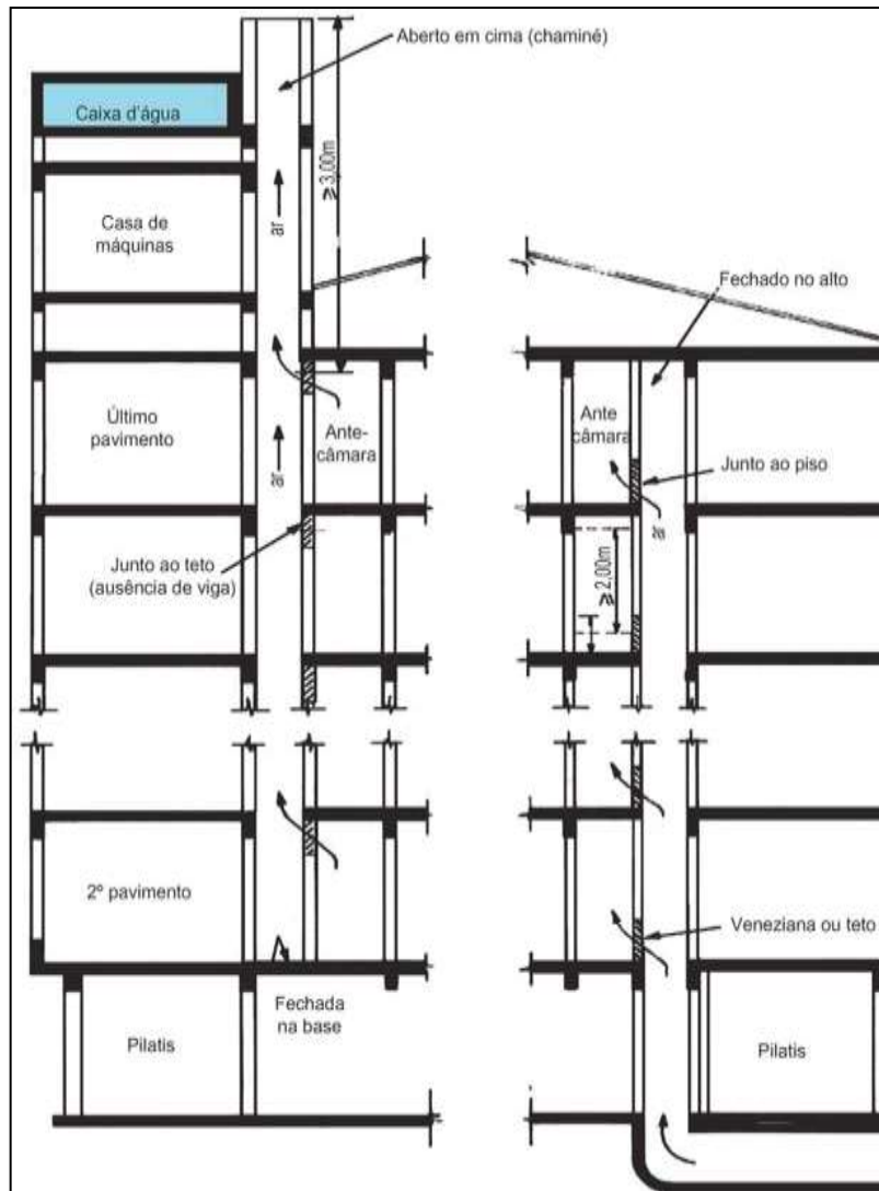
Figura 10 – Exemplo de dutos de ventilação
