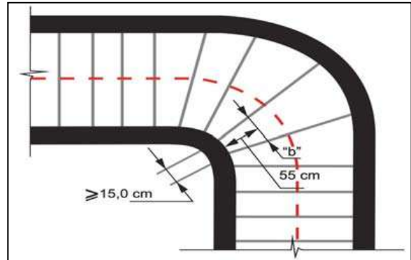
Figura 6 – Escada com laços curvos e degraus balanceados
