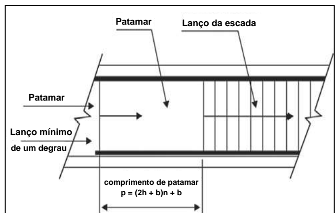
Figura 5 – Lanço mínimo e comprimento de patamar
