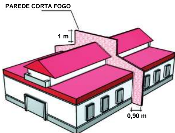
Figura 8 – Parede corta-fogo
