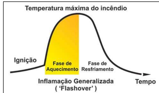
Figura 3 – Curva temperatura tempo de um incêndio
