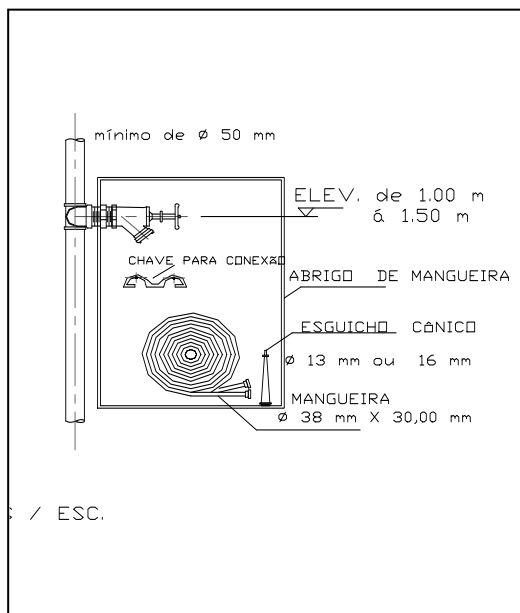
Figura 40 – Detalhe de hidrante
