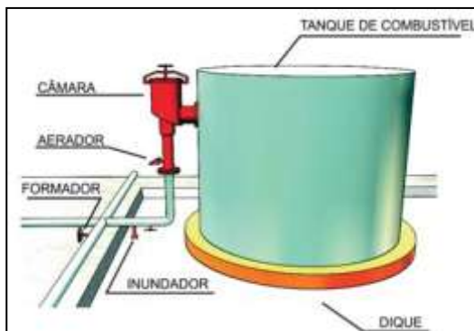
Figura 50 – Detalhe de câmara de espuma
