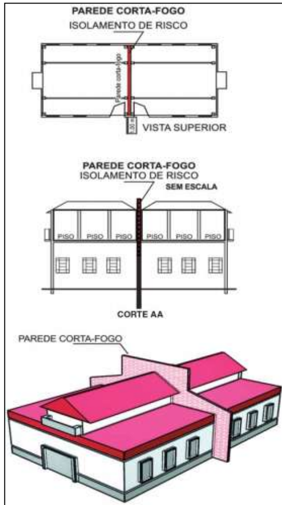
Figura 14 – Isolamento obtido por parede corta-fogo
