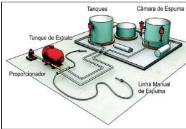
Figura 49 – Sistema semifixo
