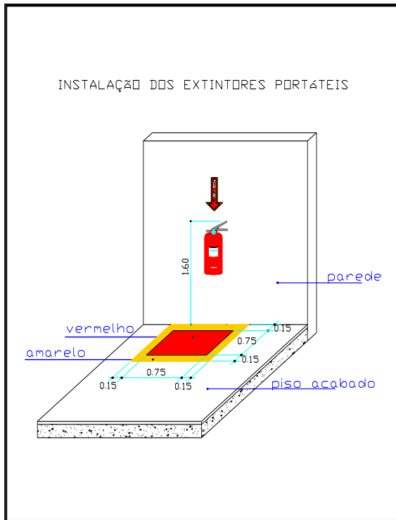
Figura 39 – Detalhe de instalação de extintores em áreas sujeitas à obstrução
