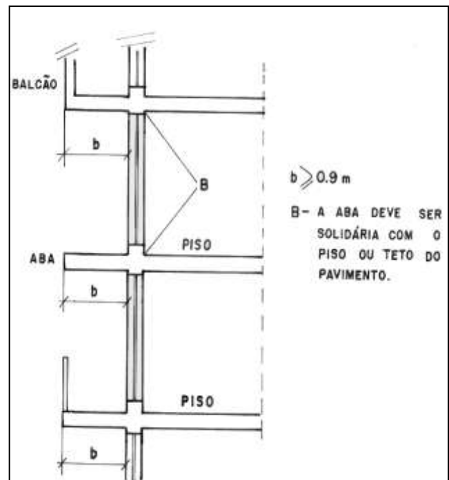
Figura 17 – Isolamento por aba horizontal ou balcão
