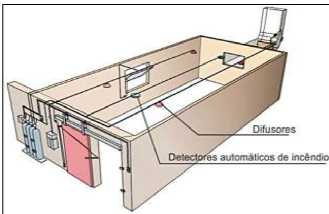
Figura 51 – Sistema de CO 2
