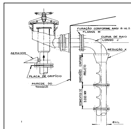
Figura 48 – Sistema fixo de espuma
