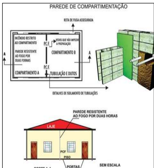
Figura 15 – Detalhes de parede de compartimentação
