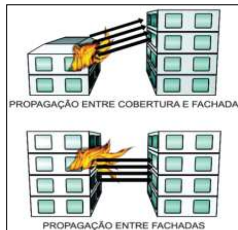
Figura 13 – Isolamento por distância de afastamento
