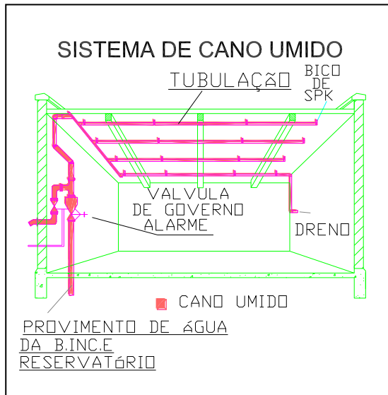
Figura 46 – Esquema de uma rede de chuveiro automático
