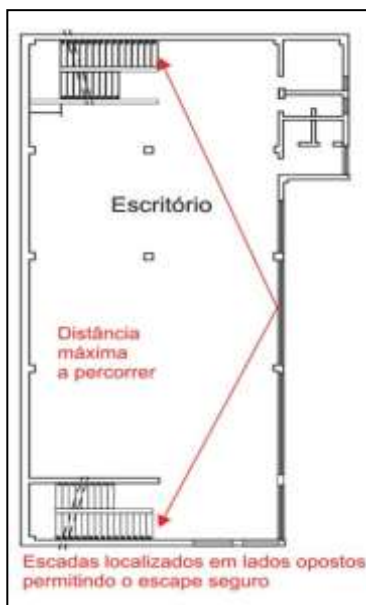
Figura 24 – Localização e Caminhamento para acesso a uma escada
