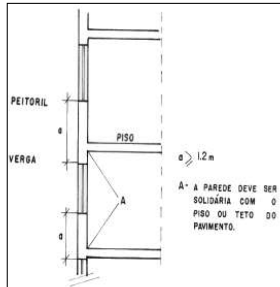
Figura 16 – Distância de afastamento entre verga e peitoril
