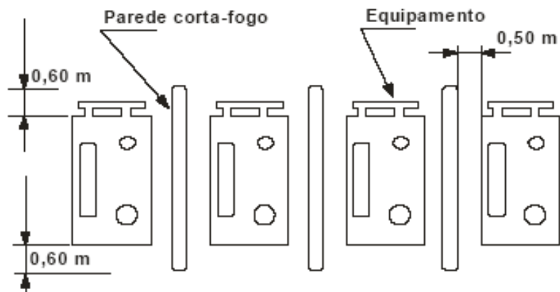
Figura 3 – Separação por parede corta-fogo
