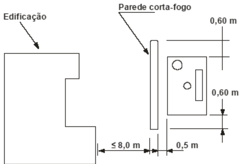
Figura 2 – Separação por parede corta-fogo
