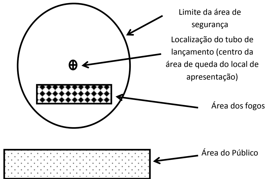
Figura 1 - Local de apresentação para tubo de lançamento na posição vertical
