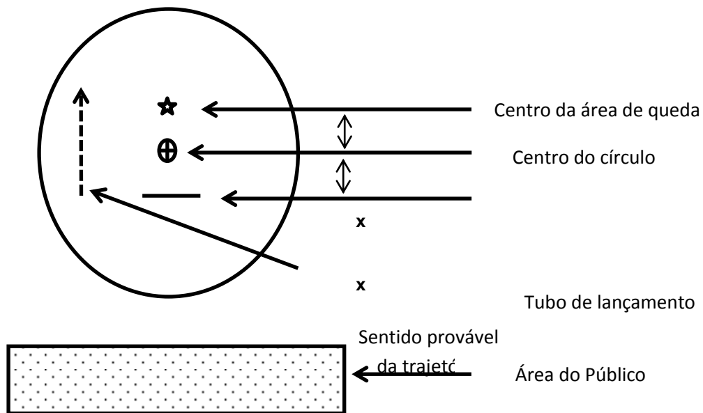
Figura 2 - Local de apresentação para tubo de lançamento inclinado
