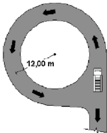
Figura 2 – Retorno circular
