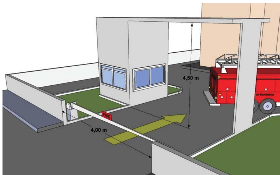
Figura 5: Largura e altura mínimas do portão de acesso à edificação
