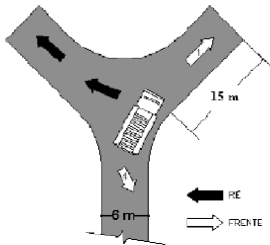
Figura 3 – Retorno em Y
